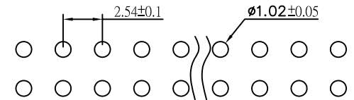
P.C.B LAYOUT
